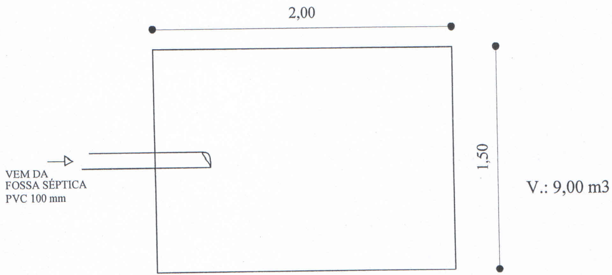
VISTA SUPERIOR
