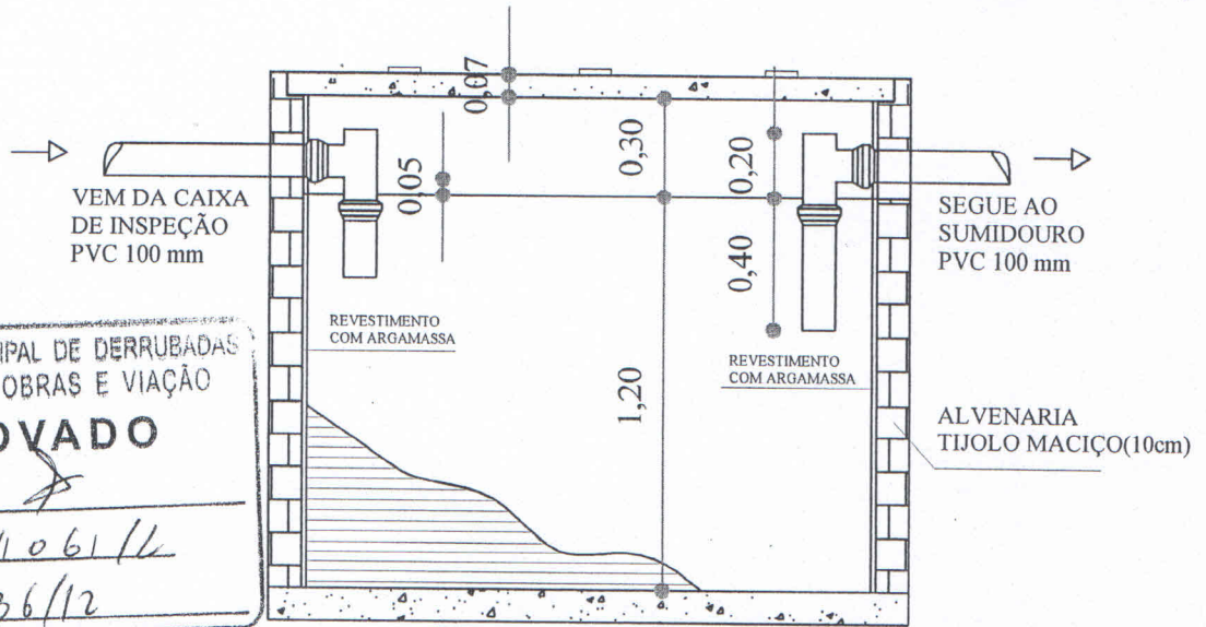
CORTE AA
