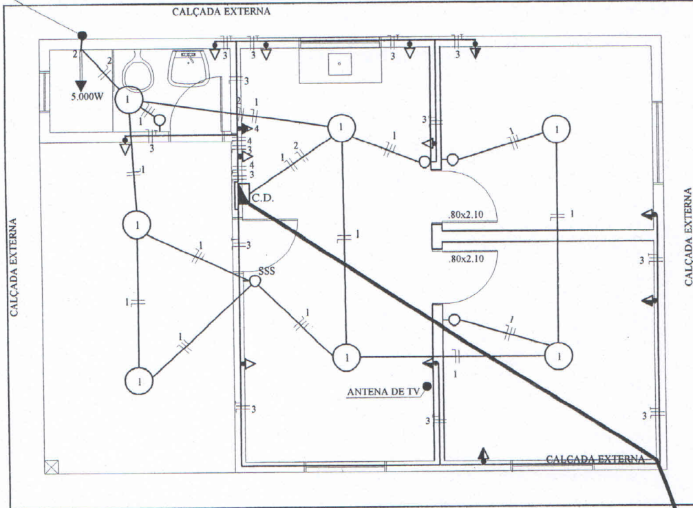
PROJETO ELÉTRICO
