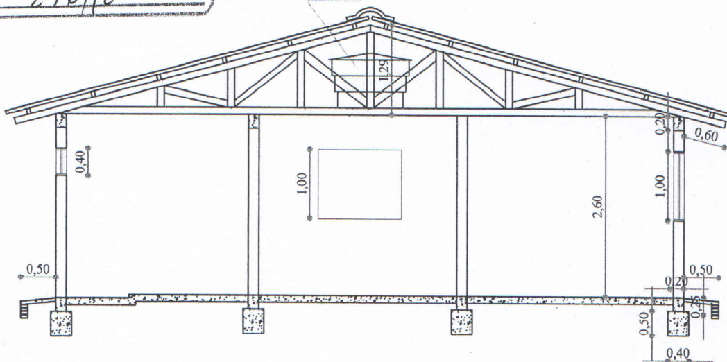
CORTE AB
